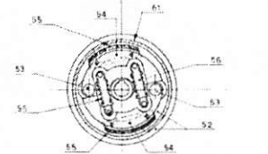
Sez. E-E
