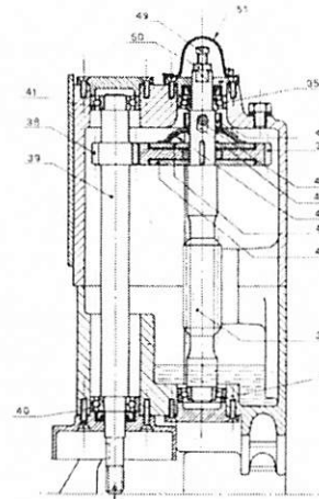
Sez. D-D
