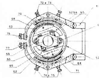
Sez. F-F
