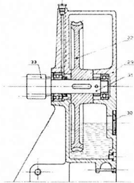
Sez. C-C
